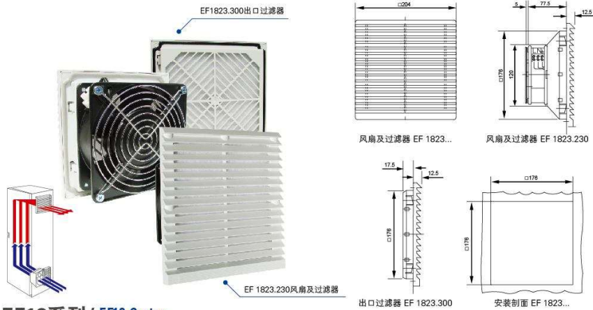
出口过滤器 EF 1823.300 安装剖面 EF 1823...
