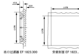
出口过滤器 EF 1823.300 安装剖面 EF 1823...
